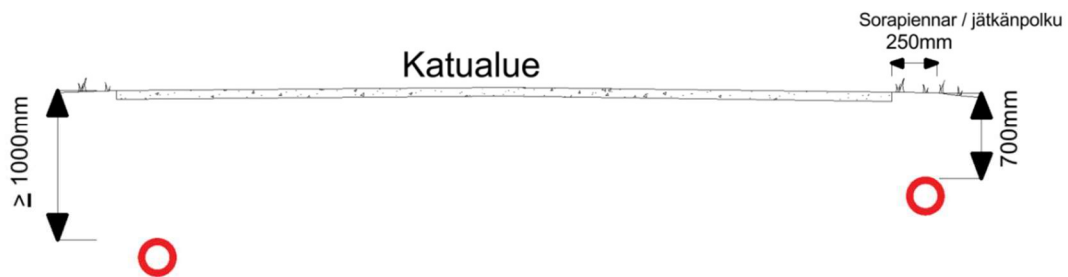
Kuva 1. Putken sijoitusyvyvydet
