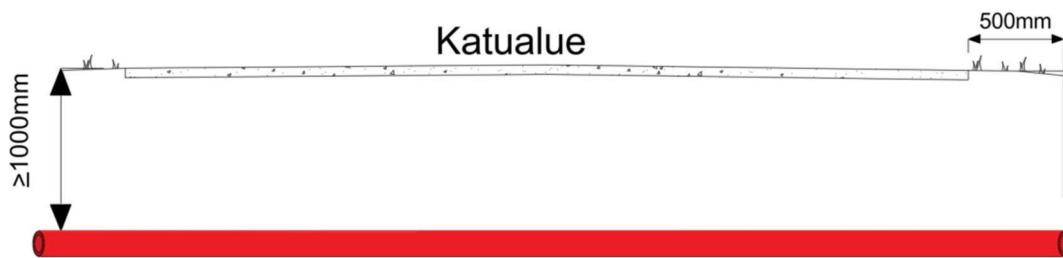
Kuva 3. Putken sijoitusvyvyys kadun alle
