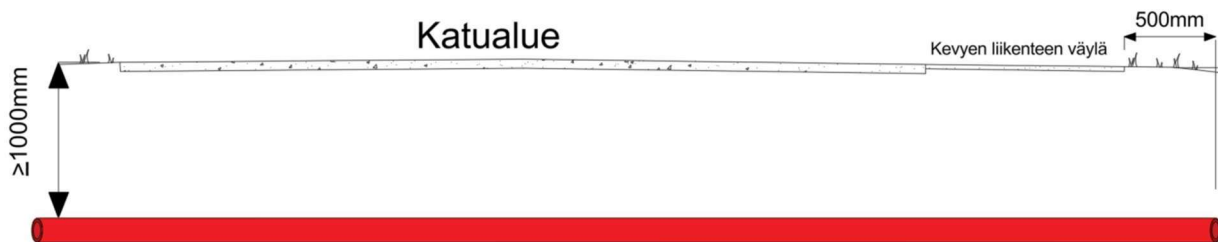
Kuva 4. Putken sijoitusvyvyys kadun sekä kevyen liikenteen väylän alle
