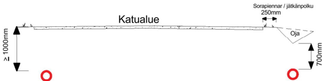
Kuva 2. Putken sijoitusyvyvydet - Putken sijoittelu ojaluiskan mukaan
