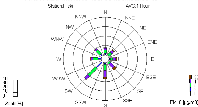
Periodic Pollution Rose Hiski 31.12.2012 24:00-31.12.2013 24:00
