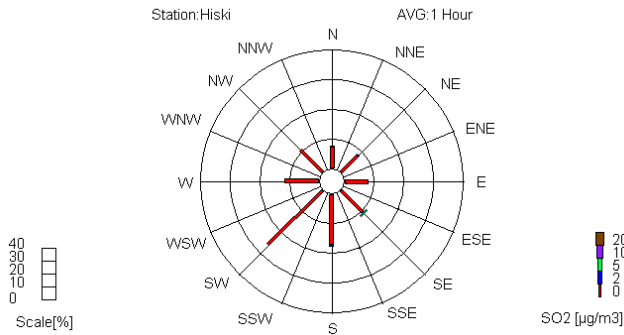
Periodic Pollution Rose Hiski 31.12.2012 24:00-31.12.2013 24:00
